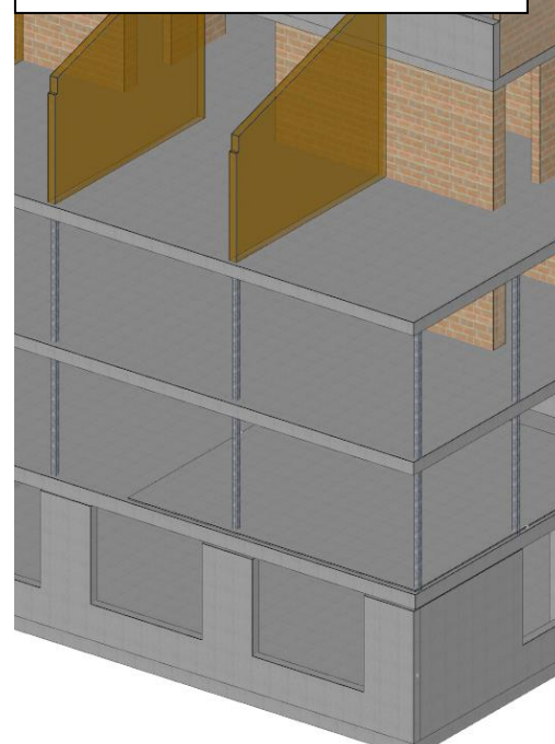
Verkleidung Stahlstützen
