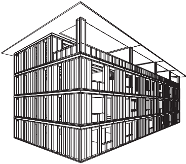
Holzrahmenbau
